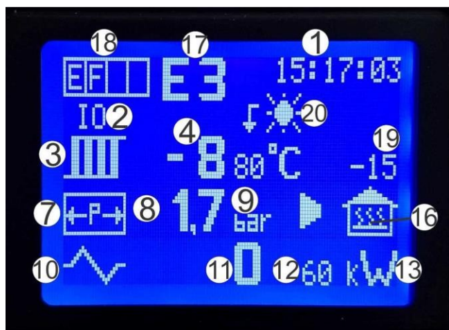
Afbeelding 8: Alle symbolen op het display van de ketel
