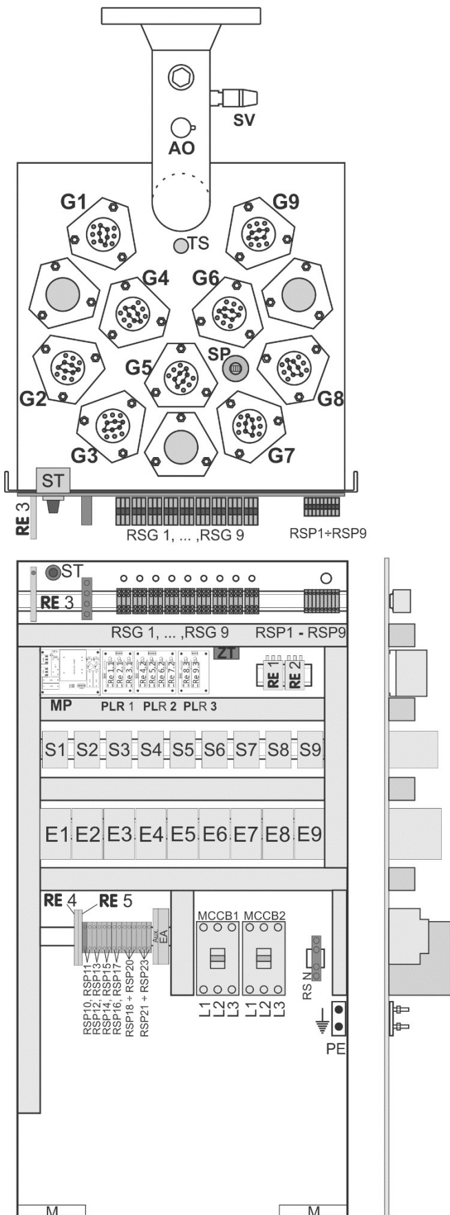
Afbeelding 14: Schakelbord en bovenplaat van het vat van ketelvermogen 180 kW
