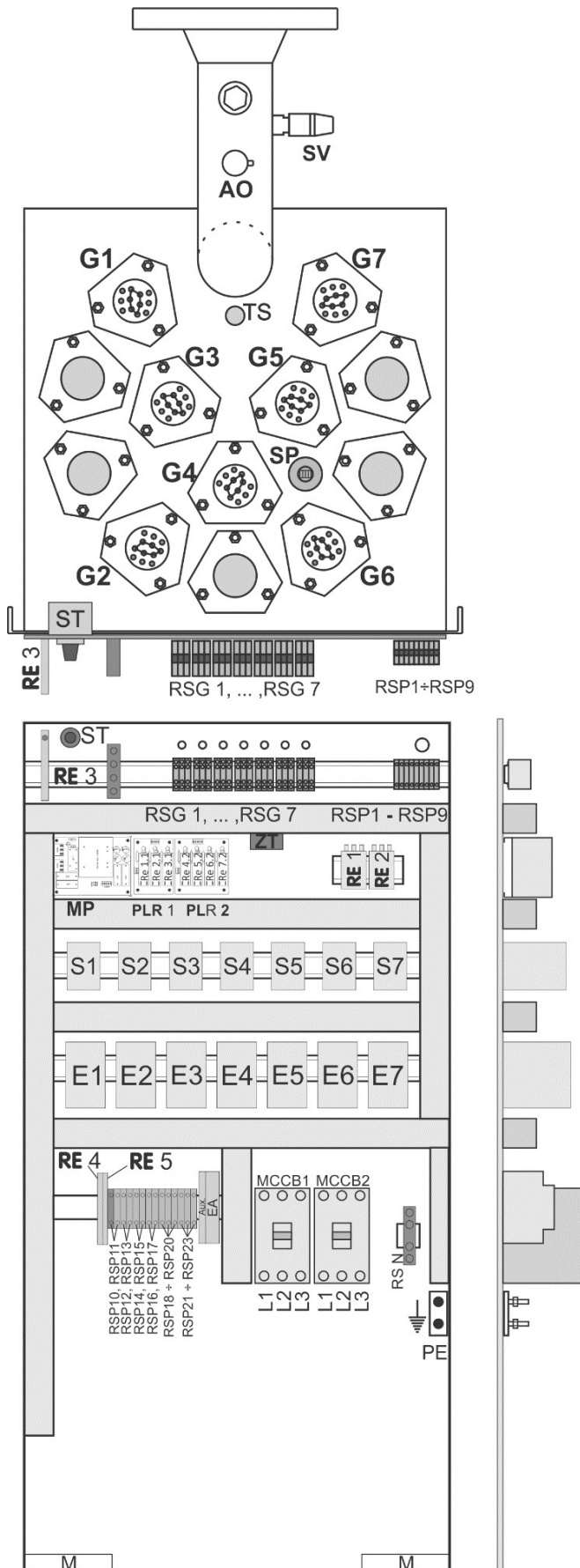
Afbeelding 12: Schakelbord en bovenplaat van het vat van
