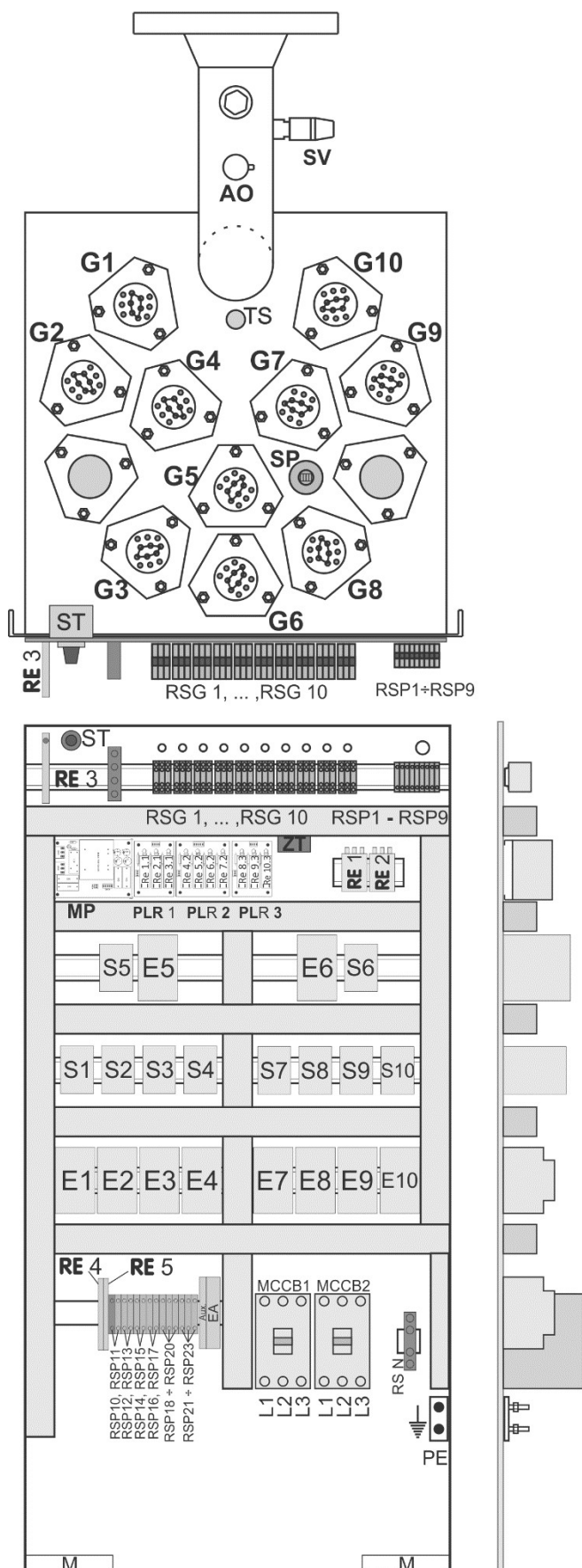
Afbeelding 15: Schakelbord en bovenplaat van het vat van ketelvermogen 200 kW
