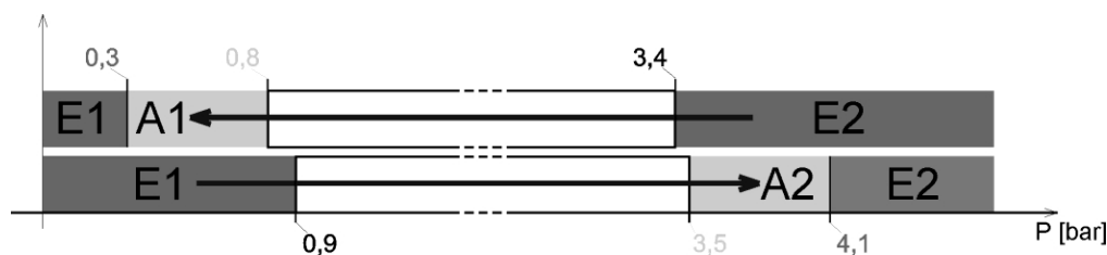
Afbeelding 9: Waarschuwingen en fouten veroorzaakt door druk
