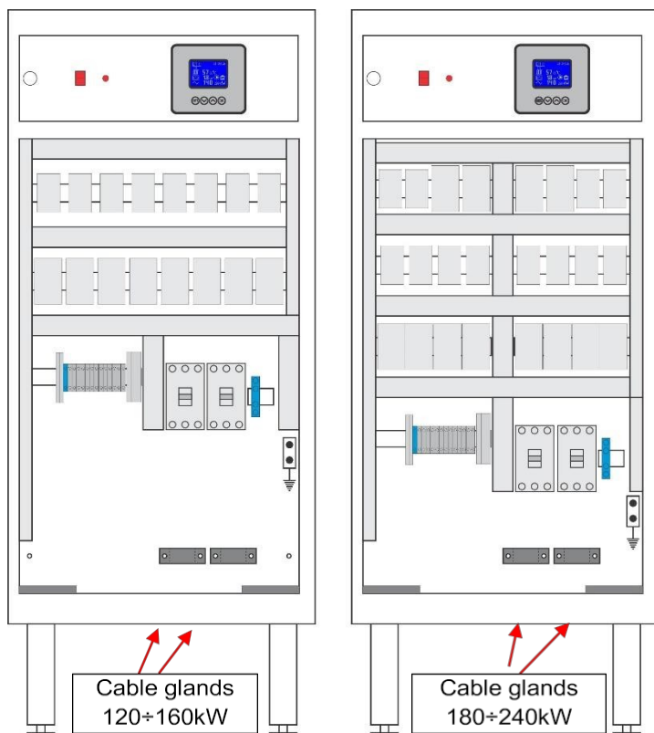
Afbeelding 6: Posities van de kabelingangen
