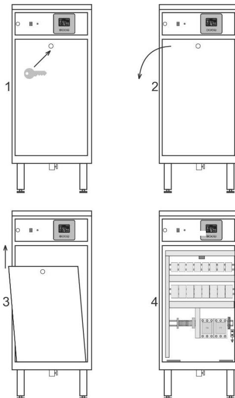
Afbeelding 4: Deur van het schakelbord demonteren
