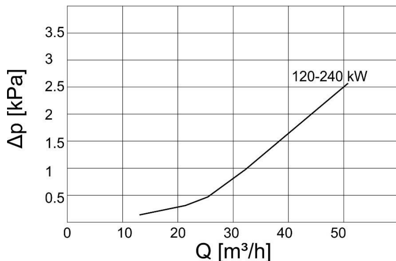
Afbeelding 2: Drukval van TK-Profesional 120 ÷ 240 kW
