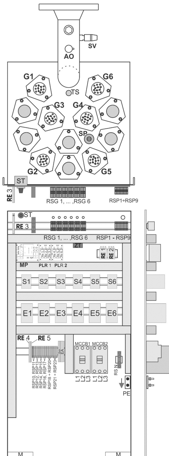
Afbeelding 11: Schakelbord en bovenplaat van een ketel met een vermogen van 120 kW
