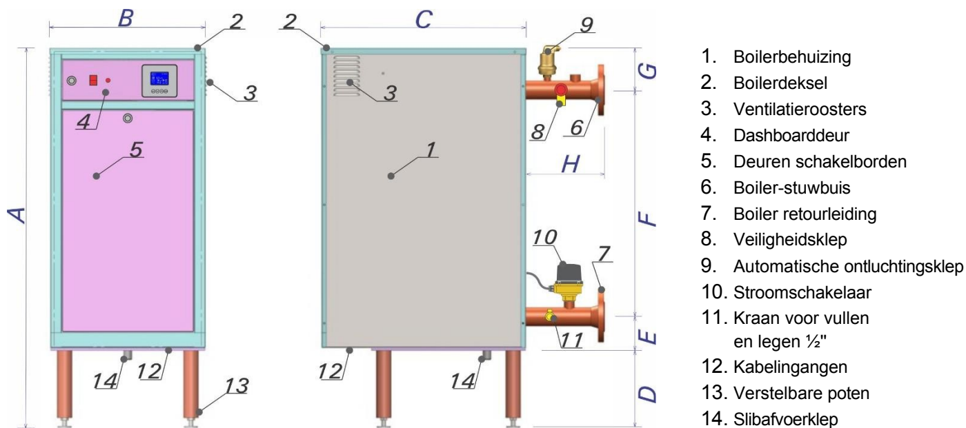
Afbeelding 1: Afmetingen en posities van TK-Profesional 120 ÷ 240 kW
