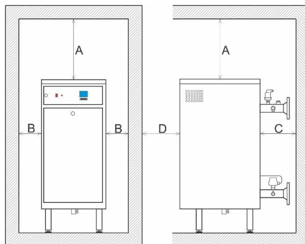
Afbeelding 3: Minimale afstand tijdens installatie
